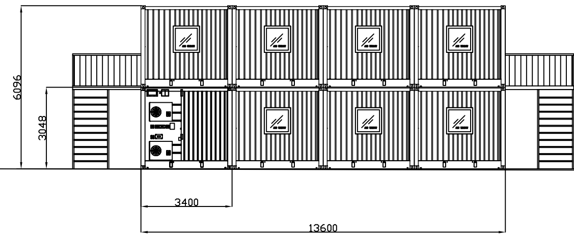
END ELEVATION
